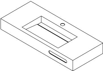
Asola rifinita portasalviette (30x4 cm) su veletta Refined tissue holder eyelet (30x4 cm) on apron Fente finie pour porte serviette (30x4 cm) sur bandeau Handtuchhalterausschnitt geschliffen (30x4 cm) im Verleimprofil
