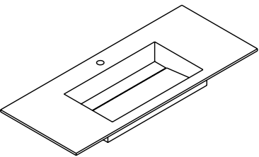
VASCA INTEGRATA SCIVOLO / BUILT-IN SLOPE SINK / VASQUE INTÉGRÉE PROFIL INCLINÉ / INTEGRIERTES BECKEN (MIT NEIGUNG)
