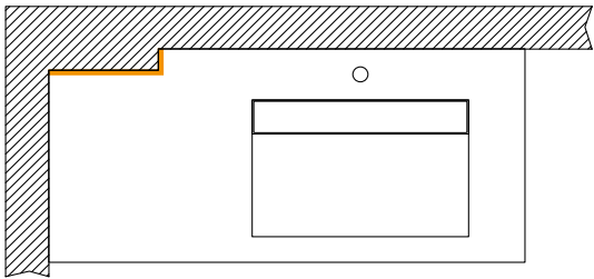
Top con scasso grezzo su lati verso il muro* Top with unfinished groove on sides towards wall Plan avec ouverture d’encastrement brute sur les côtés vers le mur Waschtischplatte mit Rohausschnitt an den wandseitigen Kanten
