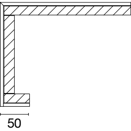
Veletta sottotop Undertop apron Bandeau sous plan de vasque Verleimprofil unter der Waschtischplatte
