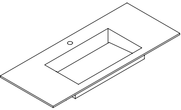
VASCA INTEGRATA FILO / BUILT-IN FLUSH SINK / VASQUE INTÉGRÉE AFFLEURANTE / INTEGRIERTES BECKEN (MIT BÜNDIGEM ABFLUSS)
