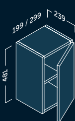
MODULE DOOR REVERSIBLE | DEPTH 24
