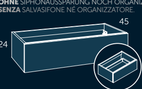
MODULE 1 DRAWER MODUL 1 SCHUBLADE MODULO 1 CASSETTO
