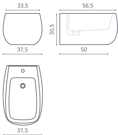
Flò suspended bidet
