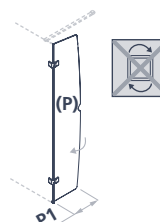
Plus Door version (02)
