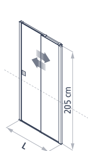
Door (02)
