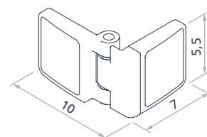
Hinge Plus Door
