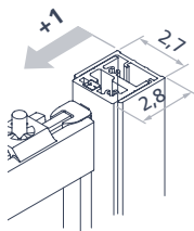
Wing door side / folding door
