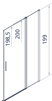
Door Plus side
