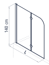
Door (01)
