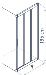
Door (02)
