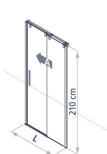
Door (02)
