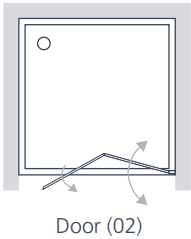
DOOR ENCUMBRANCE
