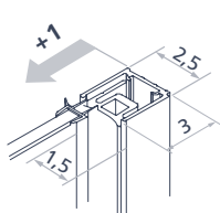
Door side
