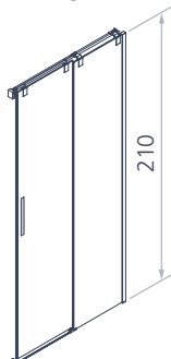
Sliding door side
