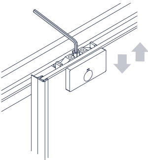
Sliding door wheels
