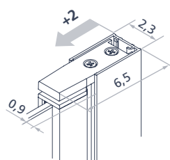
Wing door
