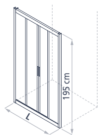
Door (02)
