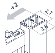
Wing door side / folding door
