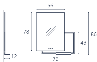
Allegro rettangolare
