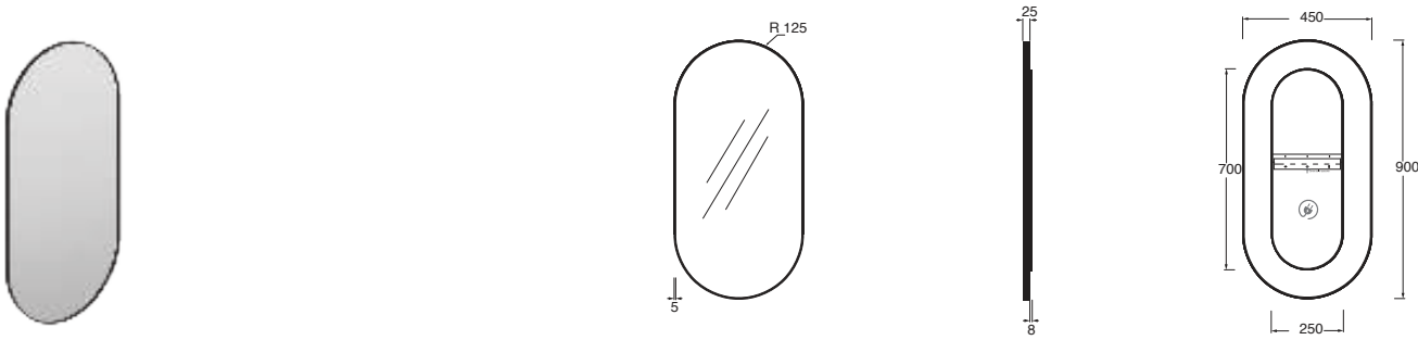
Specchio ovale 90x45 90x45 round mirror
