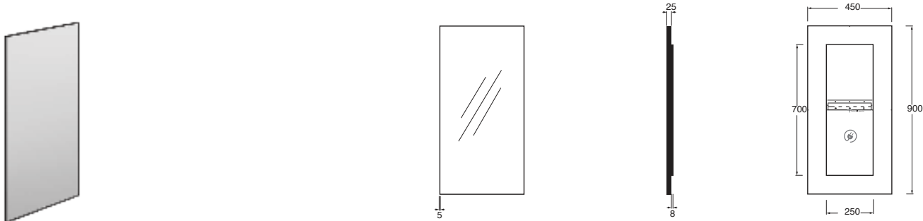
Specchio rettangolare 90x45 R90x45 rctangular mirror
