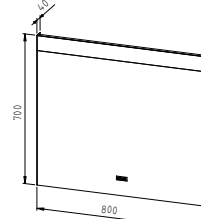
OG 80 - LED, IR, DIM, CCT, C
